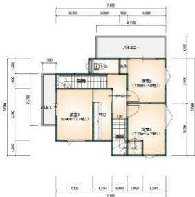
↑二階平面図
